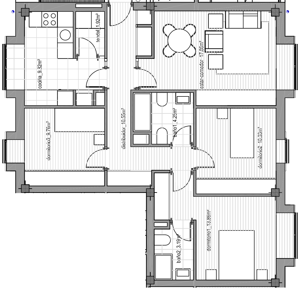
PLANTA DE DISTRIBUCIÓN VIVENDA E 1/75
