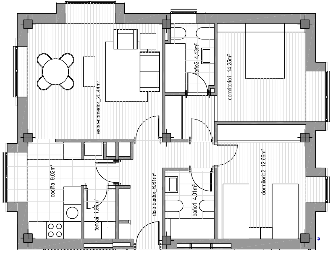
PLANTA DE DISTRIBUCIÓN VIVENDA E 1/75
