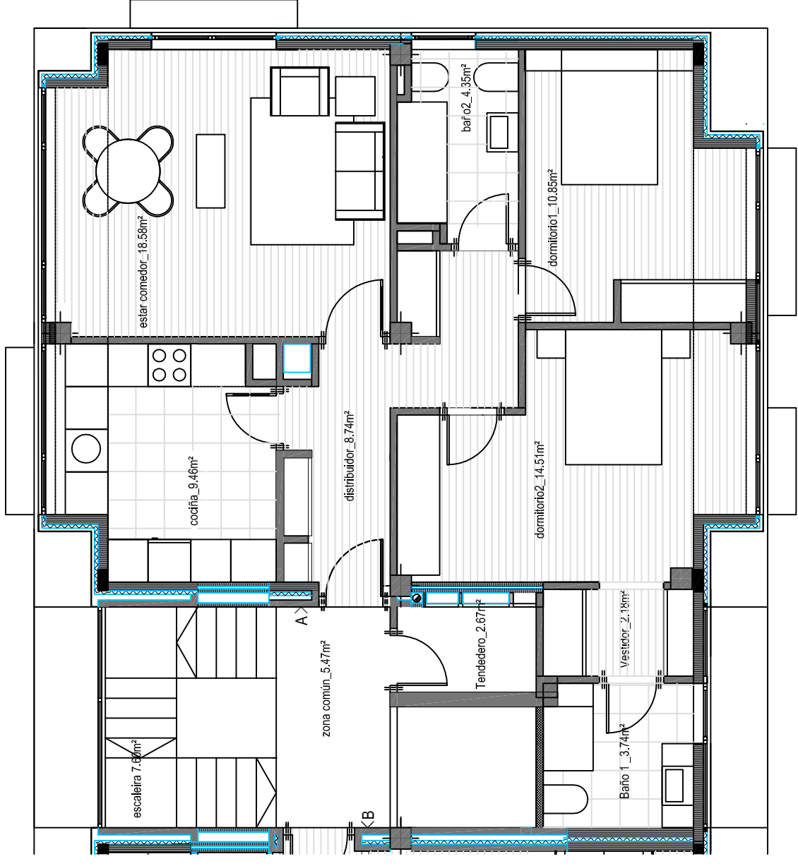
PLANTA DE DISTRIBUCIÓN VIVENDA E 1/75
